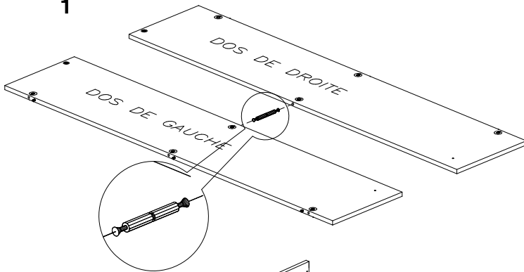
GOUJONS
